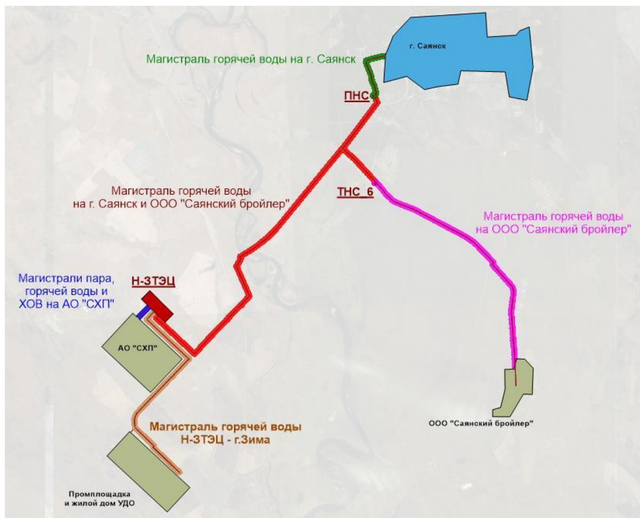
Рис. 1-2 Принципиальная схема централизованного теплоснабжения г. Саянск
