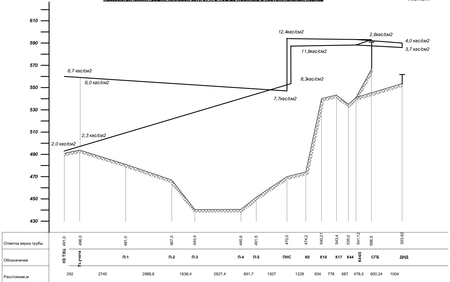
Пьезометрический график тепловой сети от Н-3 ТЭЦ до г.Саянска в неотапительный период
