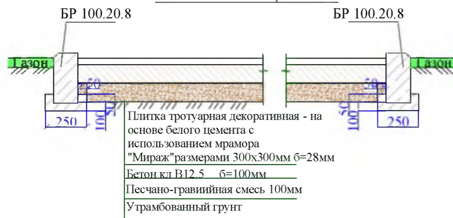
Сечение по дорожкам
